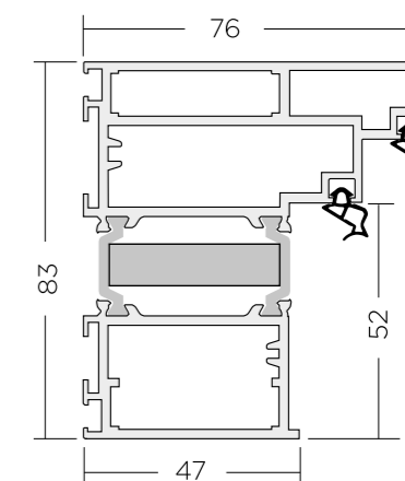
Poszerzenia Termo ALU 50mm
